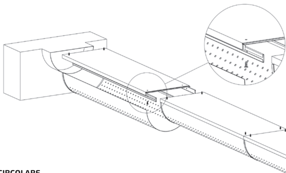
DIFFUSORE SEMICIRCOLARE
